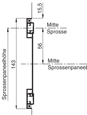
bei Standardsprosse 10 35 11
